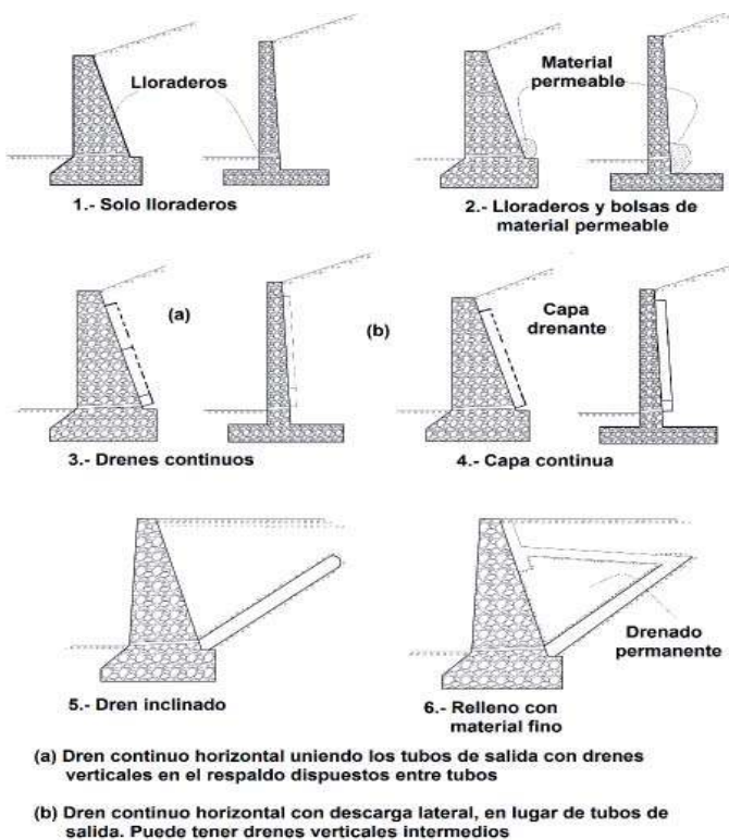
FIGURA 20 TIPOS DE MUROS
