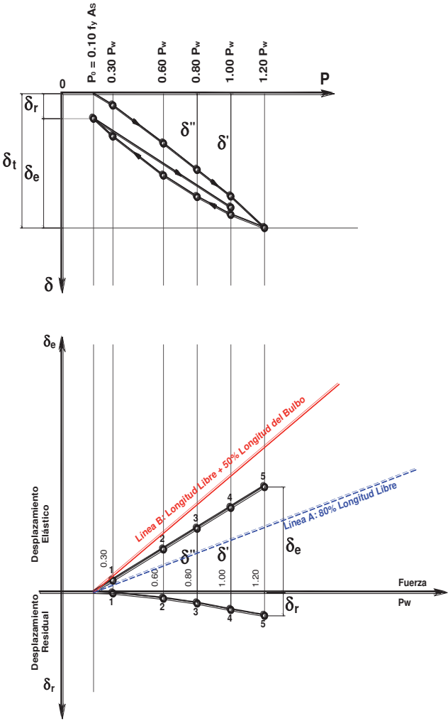
FIGURA 18 Gráficas del Ensayo de Recibimiento para Anclajes Provisionales
