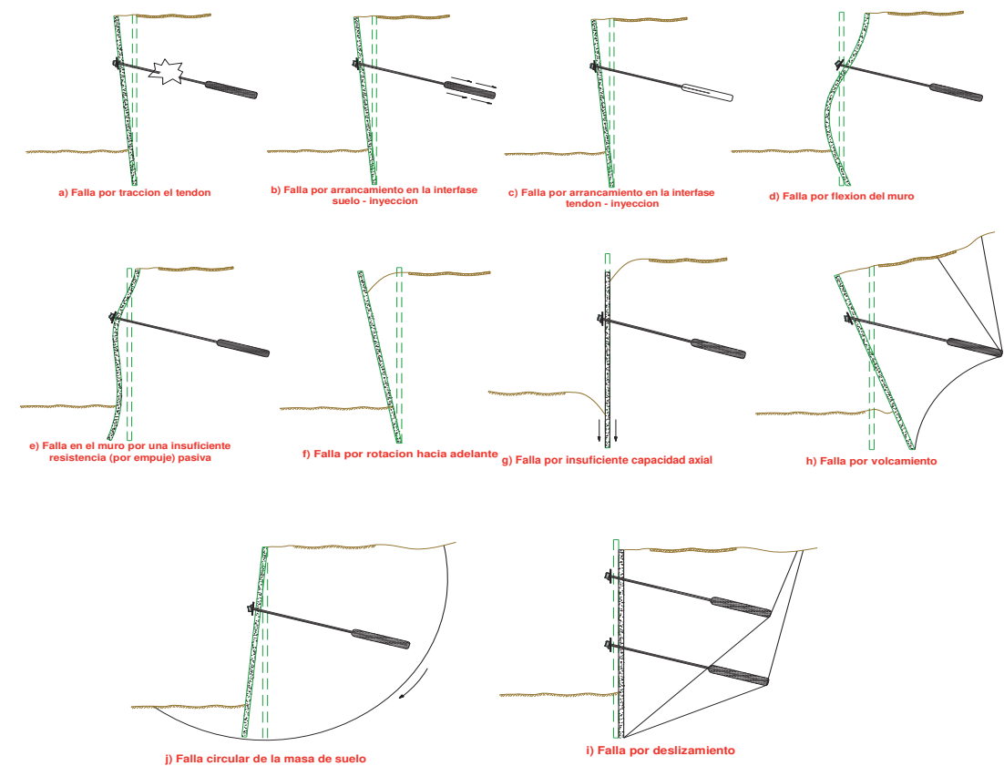
FIGURA 12 Posibles Fallas en Estructuras de Sostenimiento Ancladas
